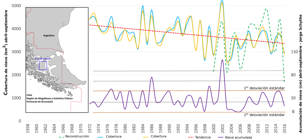
Fig. 1. Reconstrucción de la variabilidad de la cubierta de nieve en la península de Brunswick para el periodo 1972-2016 (imagen modificada de Aguirre et al. 2018).
